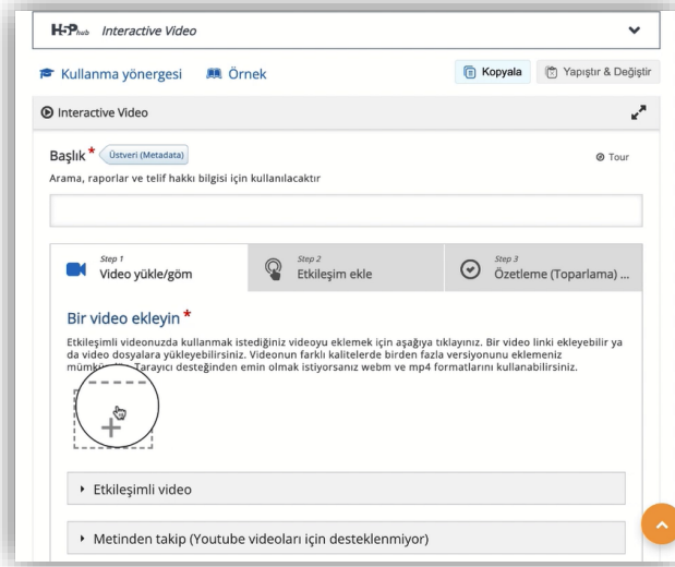
Şekil 5 Video yükleme/gömme
